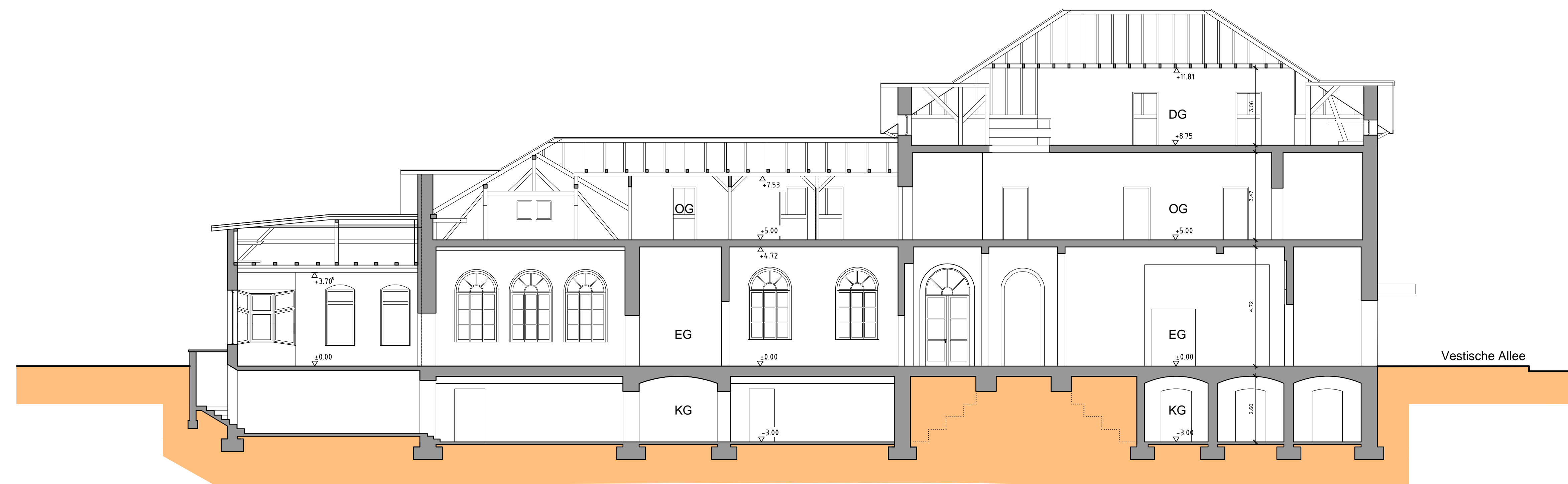
Schnitt A-A
